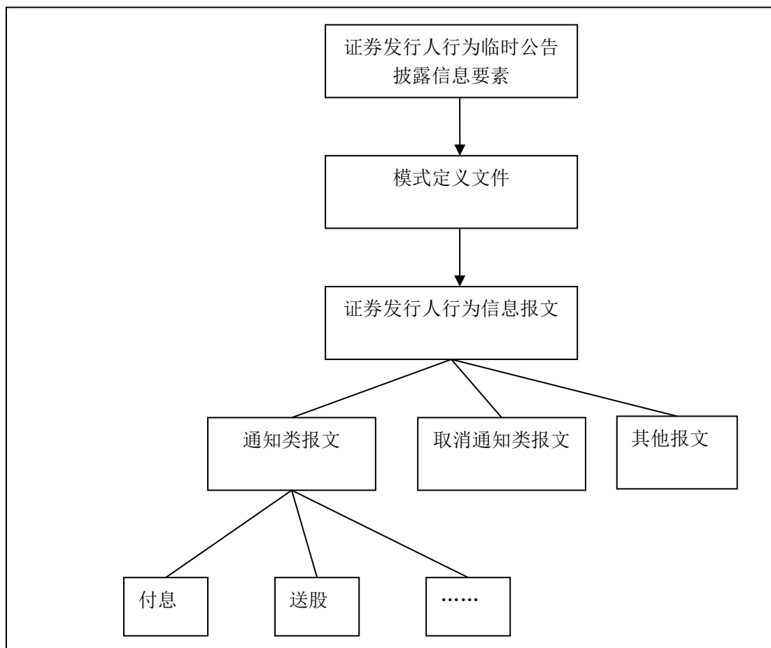
图 5 报文实例生产过程示意图
