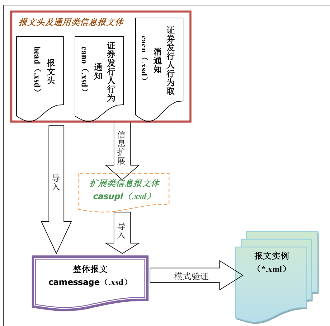
图 4 报文 XML 模式定义文件层次关系图
