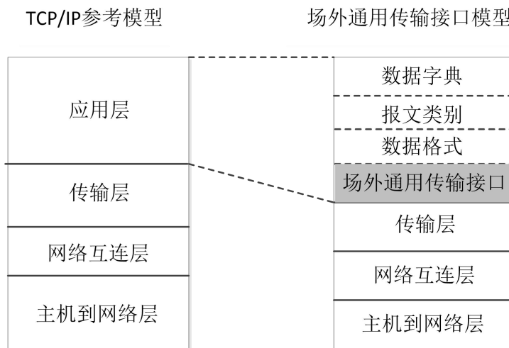
图 1 场外通用传输接口工作模型图
