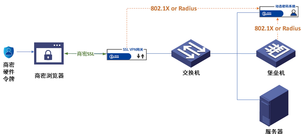
图B.1 部署方式
