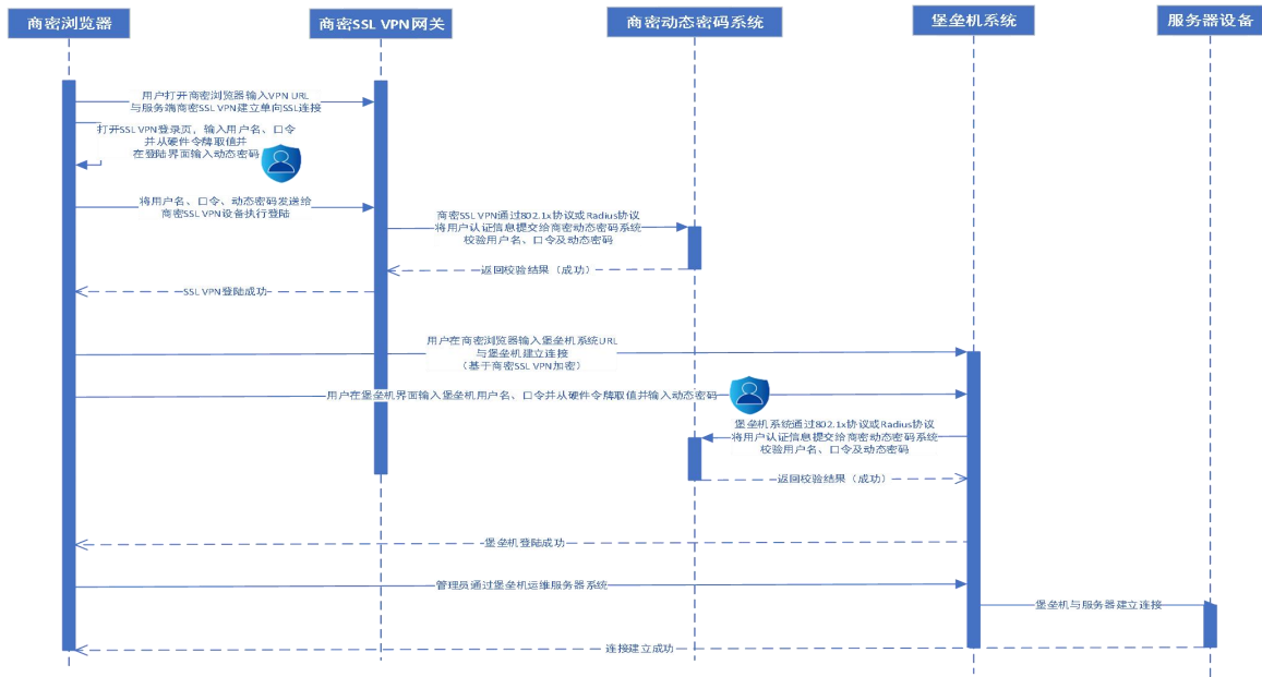
图B.2 改造后密码工作流程
